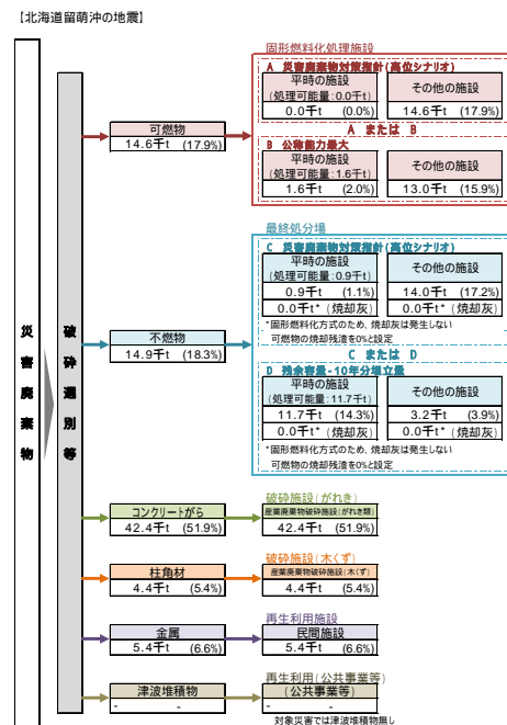
災害廃棄物処理フロー (北海道留萌沖の地震)
